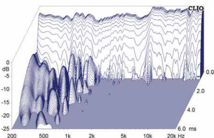
Zerfallspektrum
